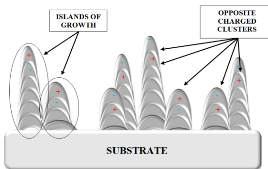
Рис. 2. Модель островкового роста пленок \text{CN}_x\text{:Eu}_y\text{O}_z
