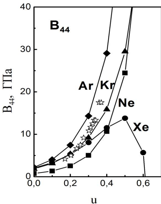
Рис.5. Залежність модулів Фукса B_{44} від стиснення u для Ne, Ar, Kr та Хе. Заповнені символи – наш розрахунок з урахуванням трьохчасткової та квадрупольної взаємодій, зірочки – експериментальне значення B_{44} для Kr.
