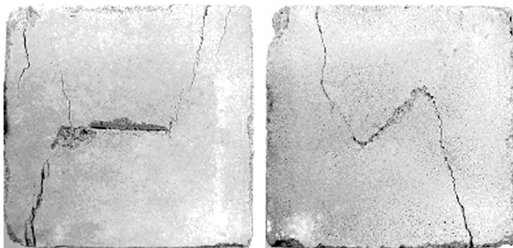
Рис. 2. Развитие трещин в образцах из ПЦМ размерами 55 \times 55 \times 20 mm с различными углами наклона \alpha начальных сквозных трещин при их осевом сжатии: a – \alpha = 0 , б – \pi/4
