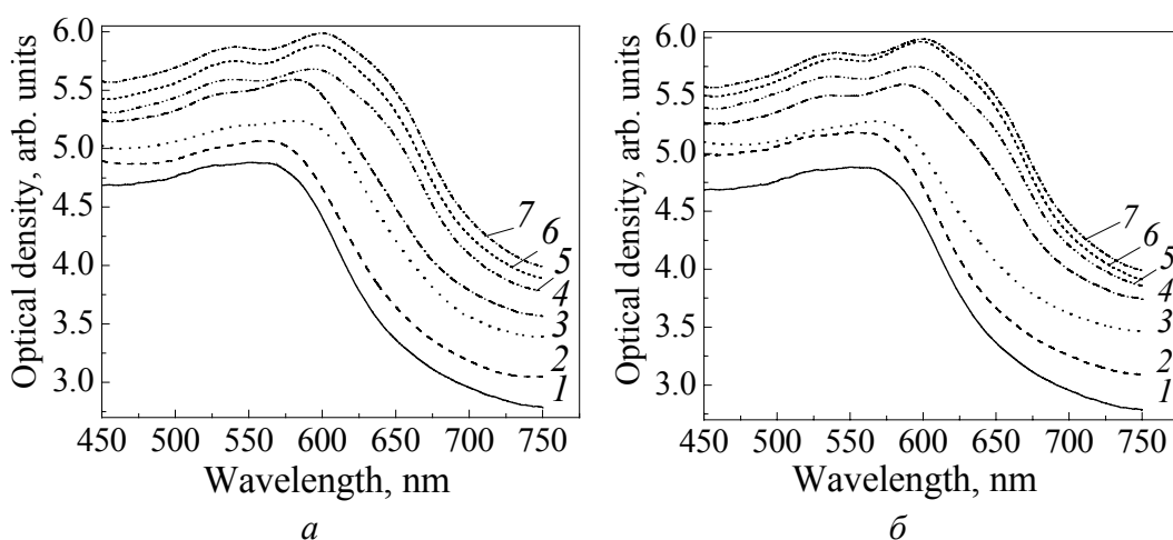
Рис. 1. Спектры поглощения \text{Fe}(\text{phen})_2(\text{NCS})_2 при комнатной температуре и повышении (а) и понижении (б) давления, GPa: а: 1 – 0, 2 – 0.279, 3 – 0.401, 4 – 0.618, 5 – 0.931, 6 – 1.355, 7 – 1.814; б: 1 – 0, 2 – 0.138, 3 – 0.393, 4 – 0.509, 5 – 0.779, 6 – 1.201, 7 – 1.814
