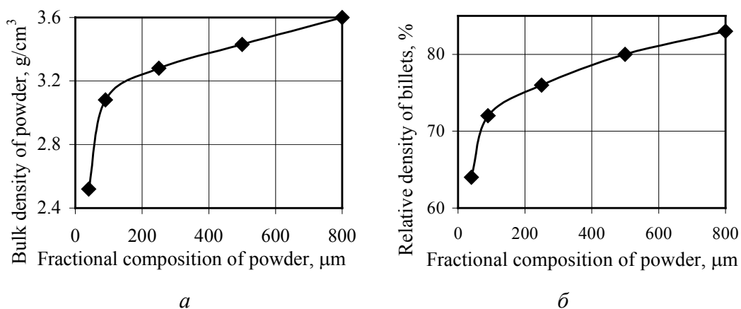
Рис. 1. Зависимость насыпной плотности порошка (а) и относительной плотности заготовок после гидростатической обработки (б) от фракционного состава порошка Р6М5Ф3
